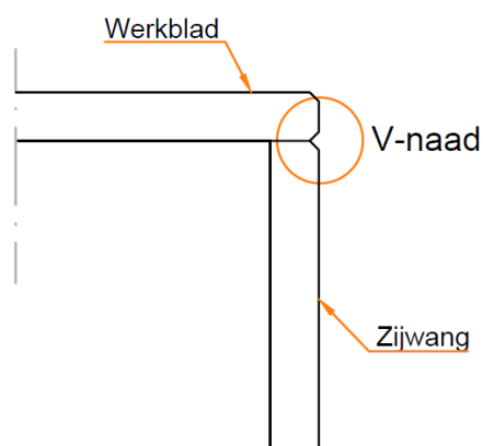
Detail Randafwerking V-naad t.b.v. aansluiting werkblad op stollenwand
